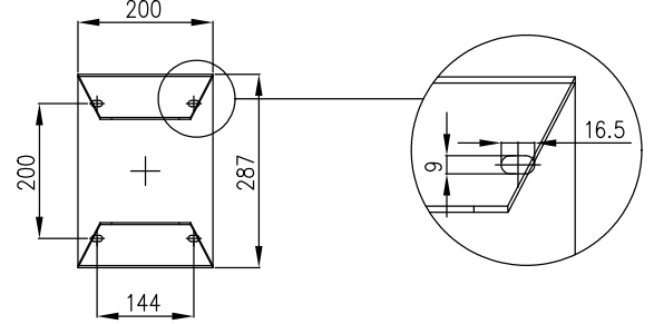
MONTAJ DETAYLARI
